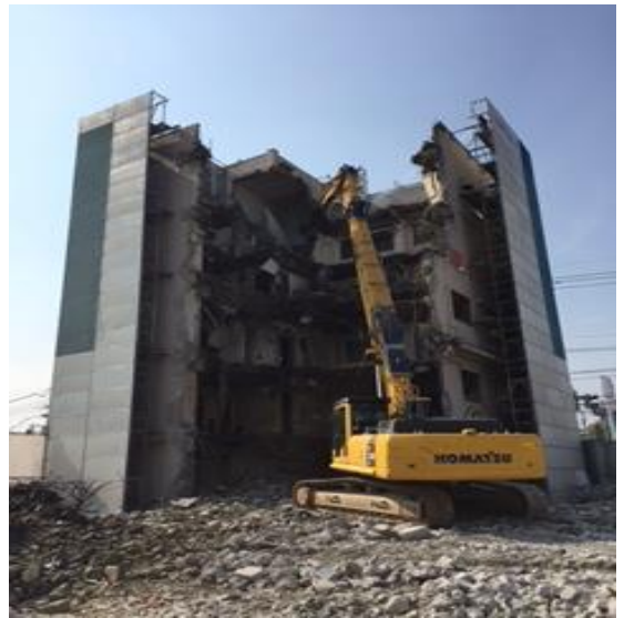
建屋解体
